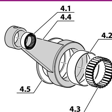
2° STADIO - 2nd STAGE 16-00-0101/R
