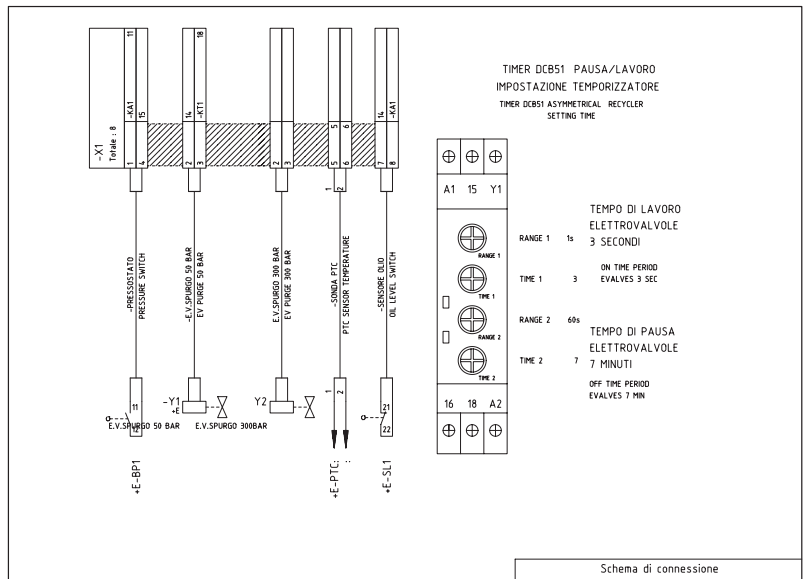
Schema di connessione
